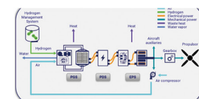
[항공용 연료전지 시스템 개념도(예시)]
