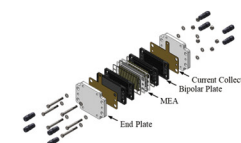
[연료전지 스택 조립도(예시)]
